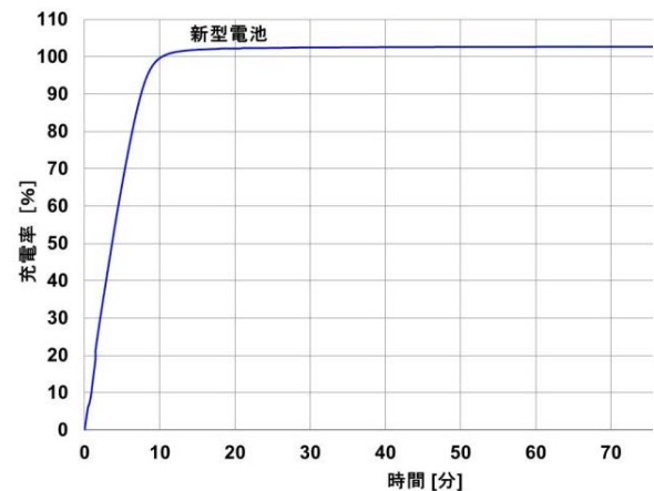
新型リチウムイオン電池の充電曲線（環境温度：25℃）
