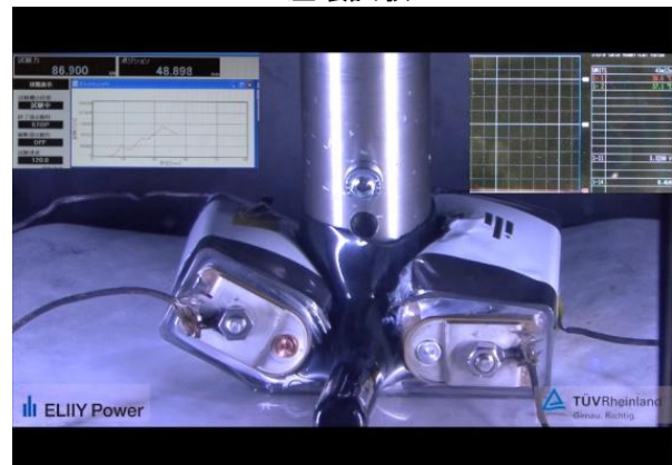
圧壊試験
